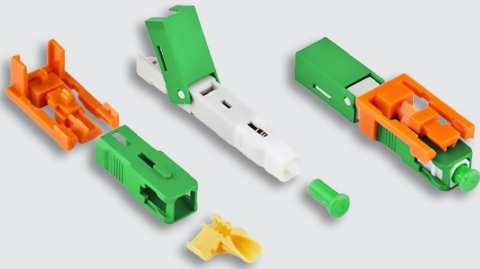
LX-14(52mm)-APC
