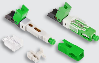
LX-09-B(52mm)-APC
