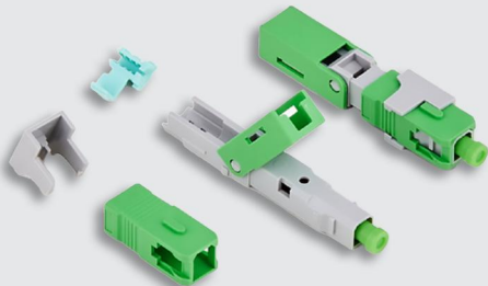
LX-11-B(52mm)-APC
